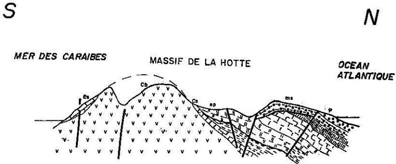
Figure 4. Coupe géologique de la Grande Anse
