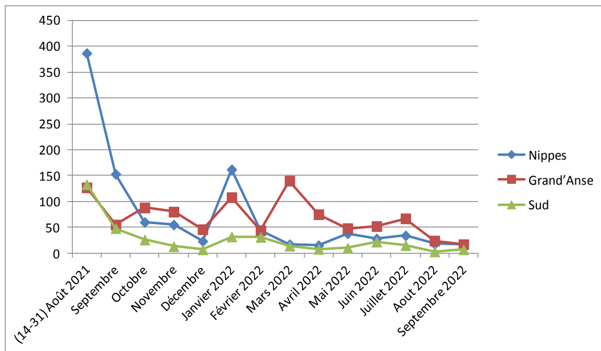
Figure 2. Courbes évolutives des séismes enregistrés dans les Nippes, la Grand'Anse et le Sud du 14 août 2021 au 30 septembre 2022.
