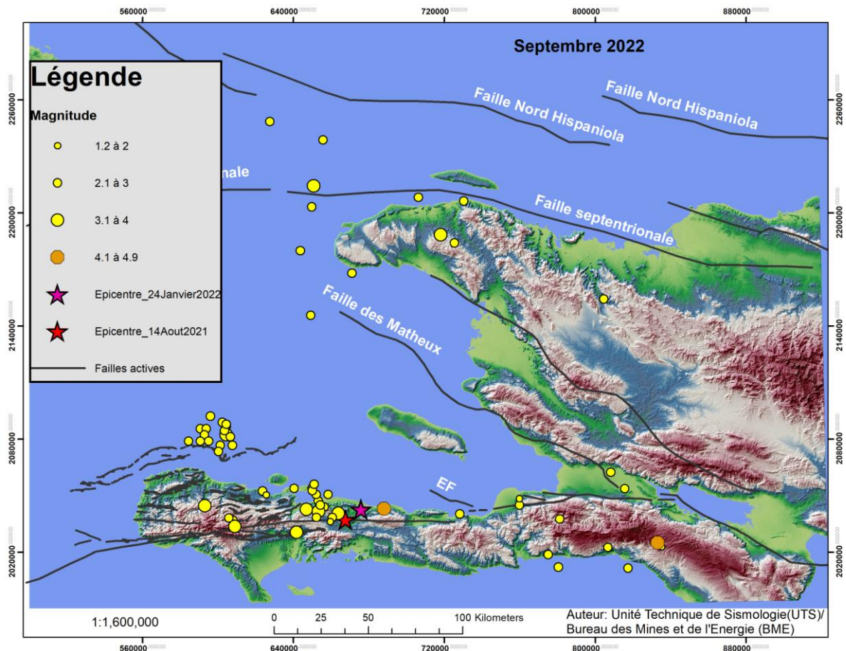
Figure 1. Cartes des epicentres des séismes enregistrés au cours du mois de septembre 2022
